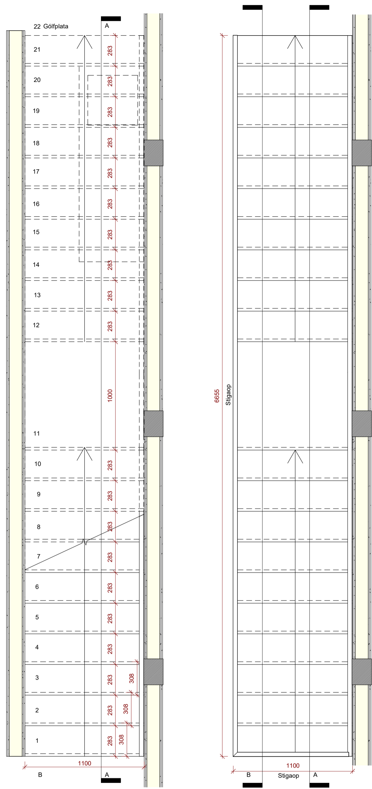
Grunnmynd stiga 1 : 20
