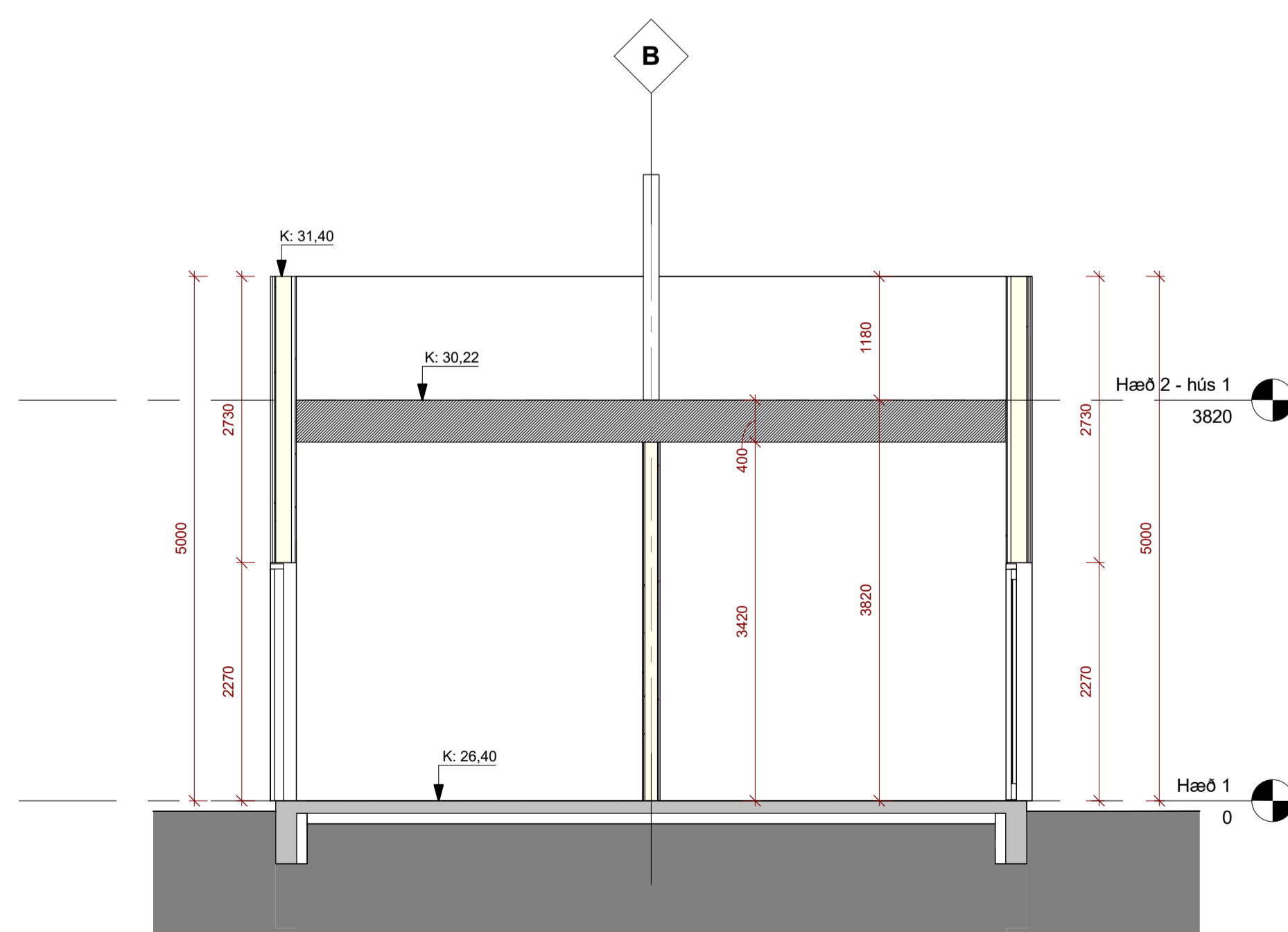
Snið D 1 : 50
