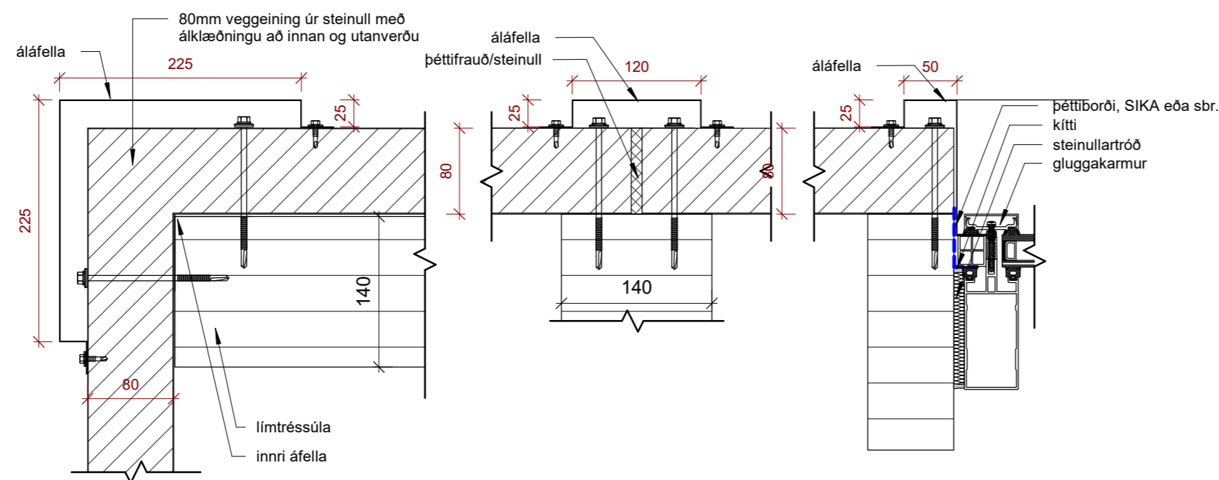
Frágangur við úthorn
