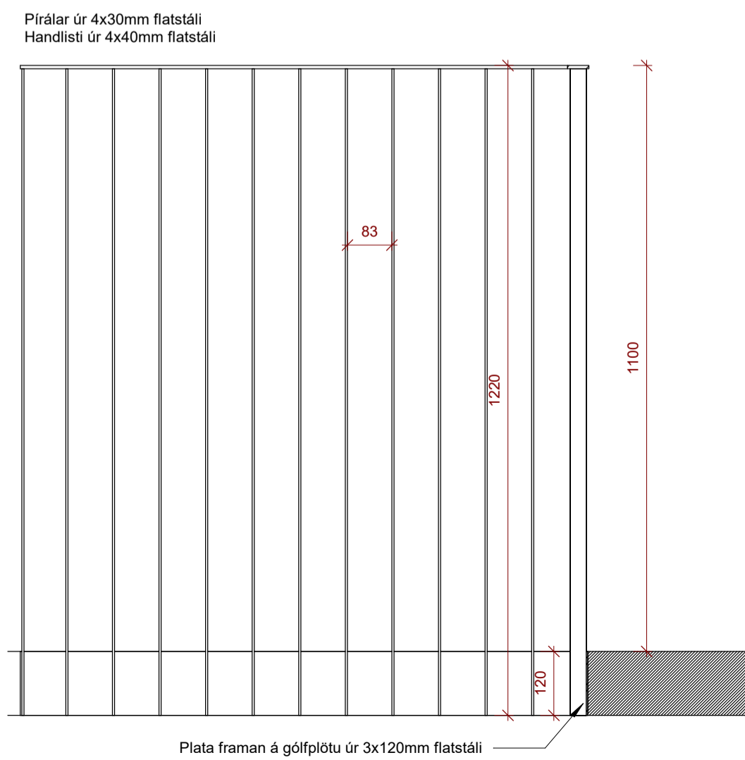
Snið/hlutaámynd á handrið á millilofti 1 : 10
