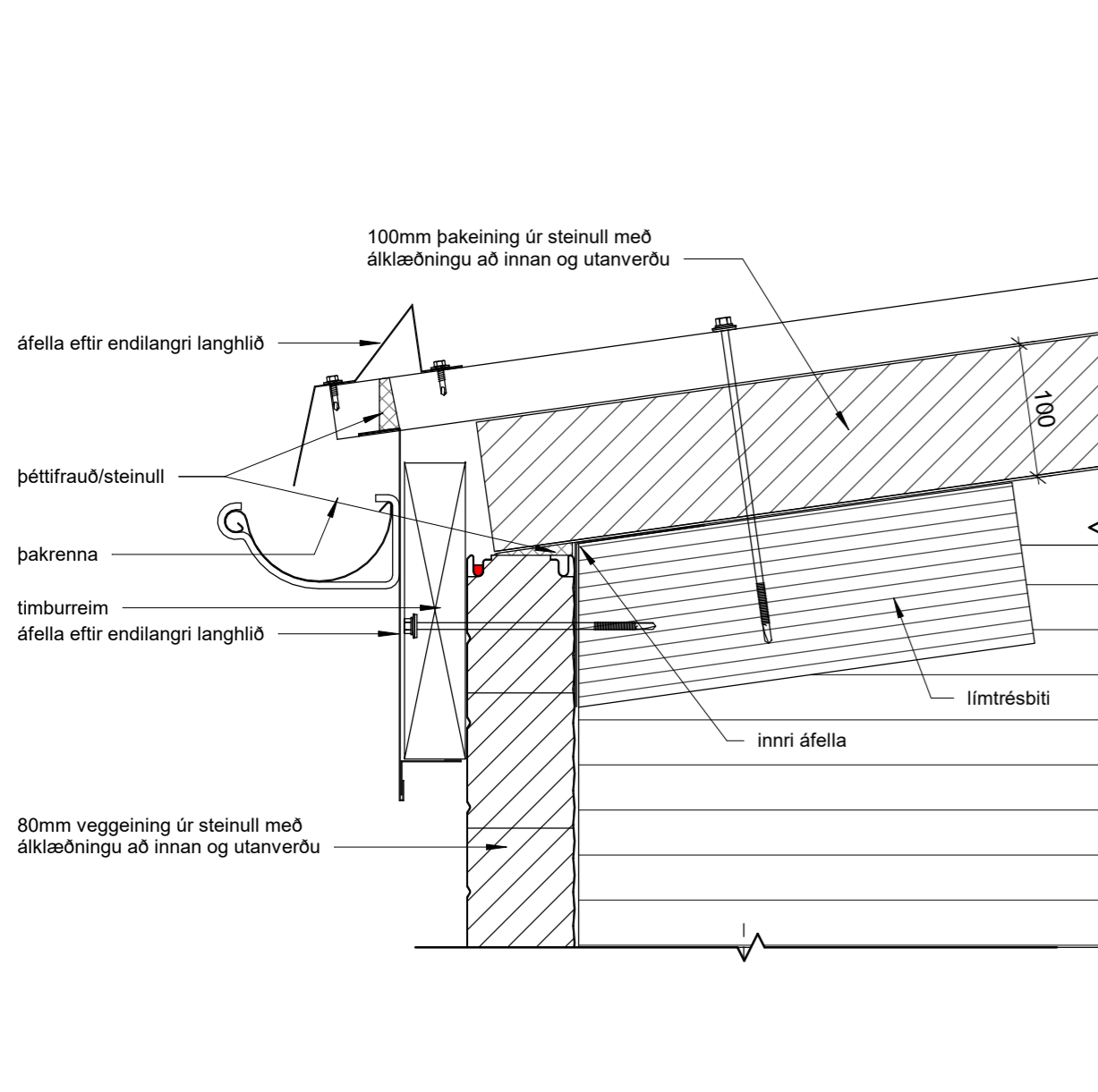
Frágangur við þakbrún
