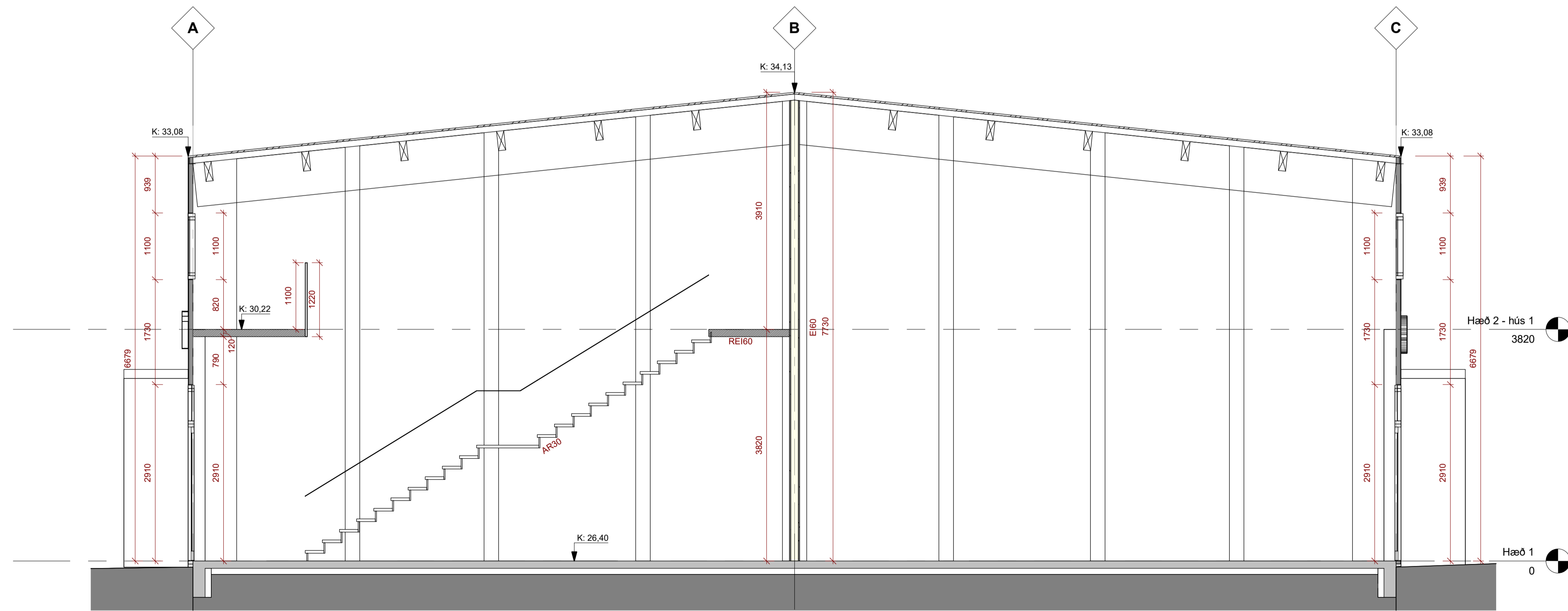
Snið B 1 : 50
