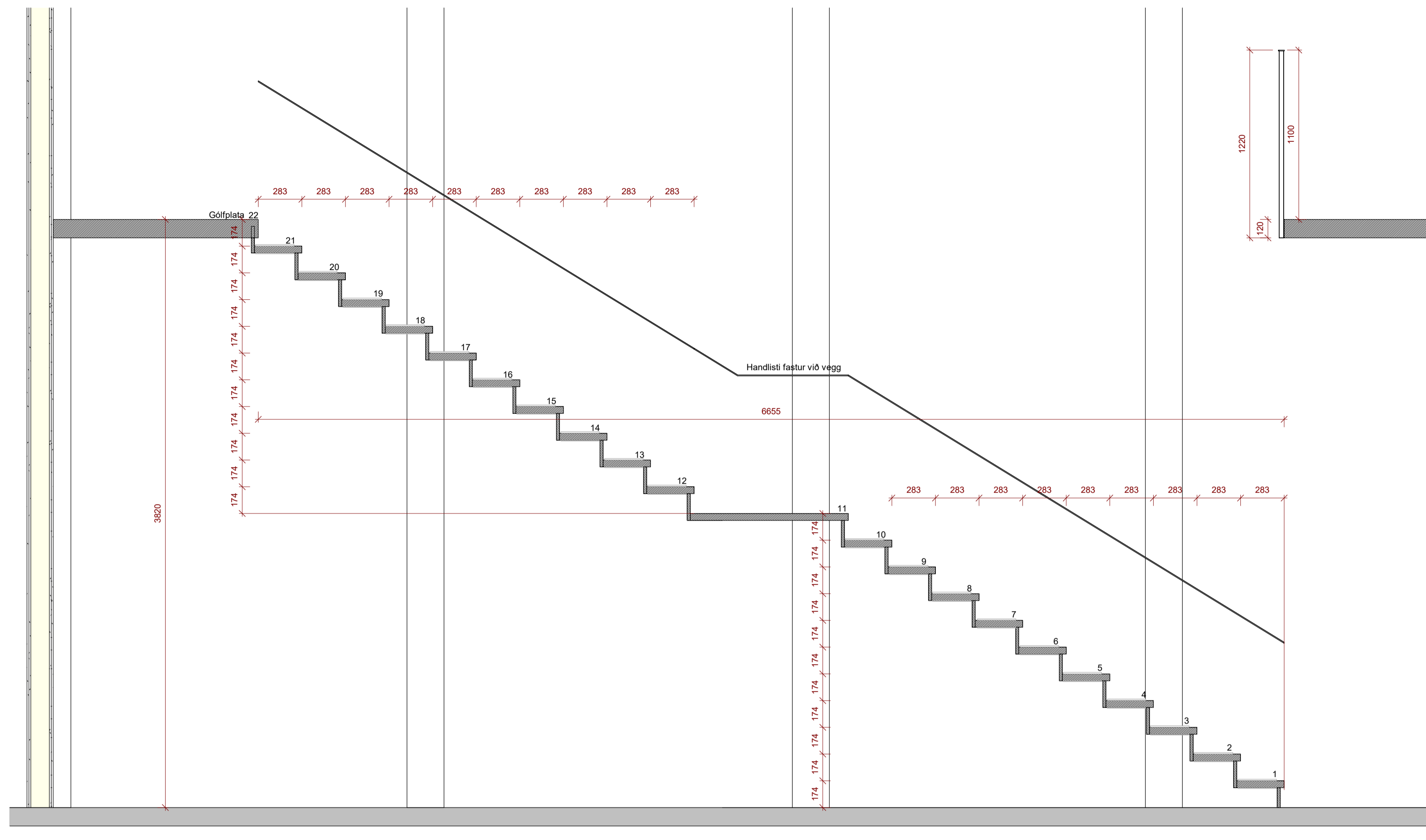
Snið A í stiga 1 : 20
