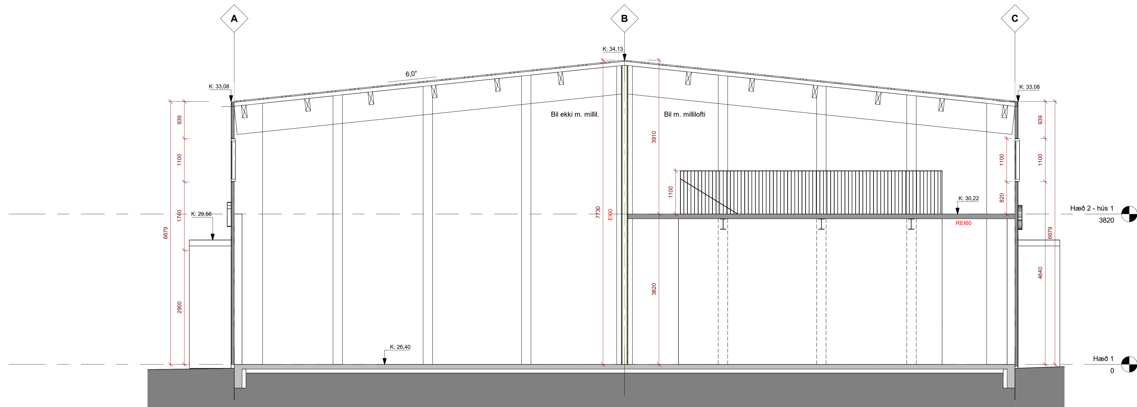
Snið A 1 : 50
