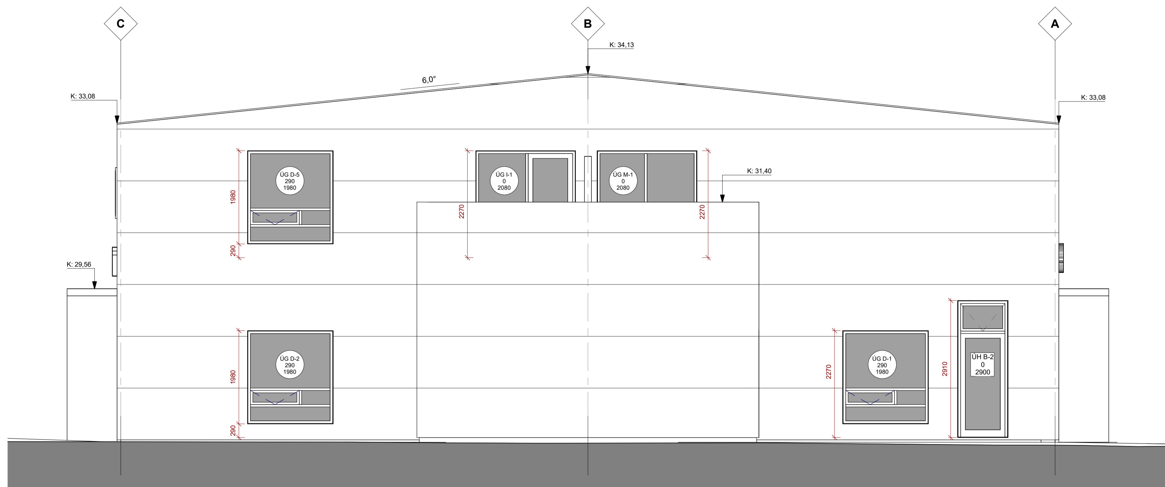
Ásýnd norður 1 : 50
