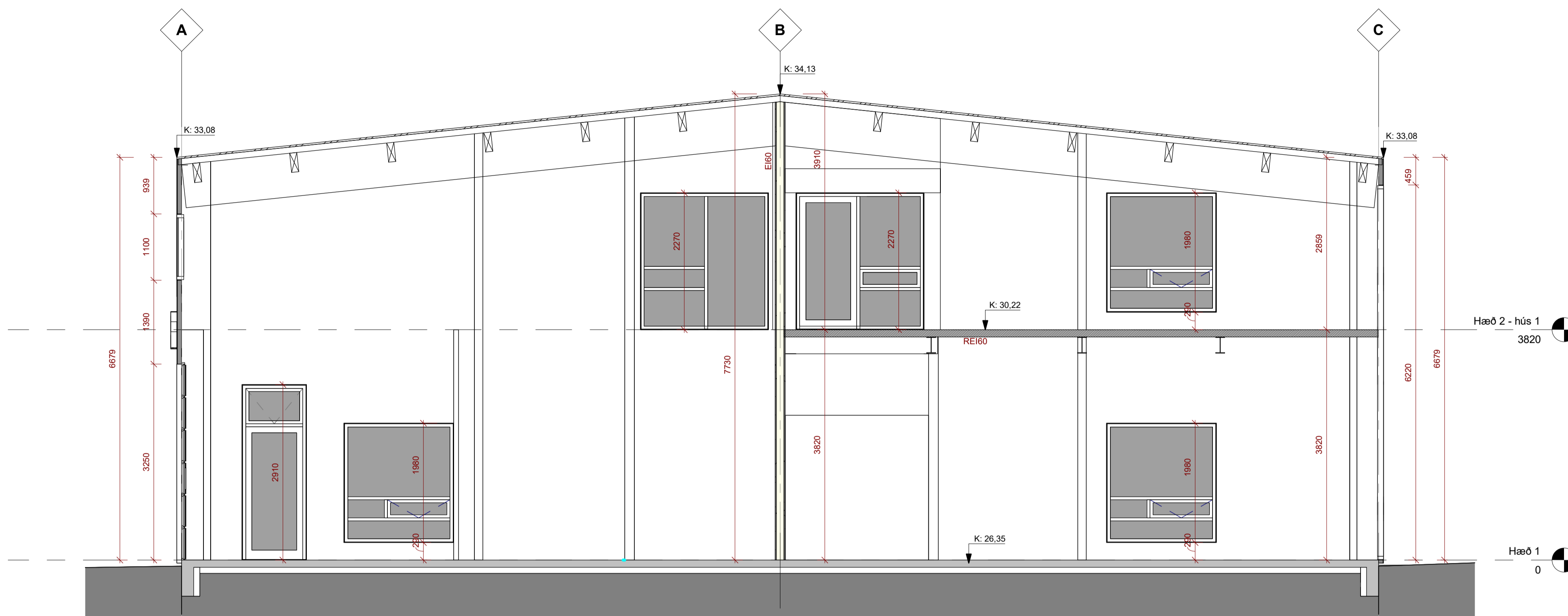
Snið C 1 : 50
