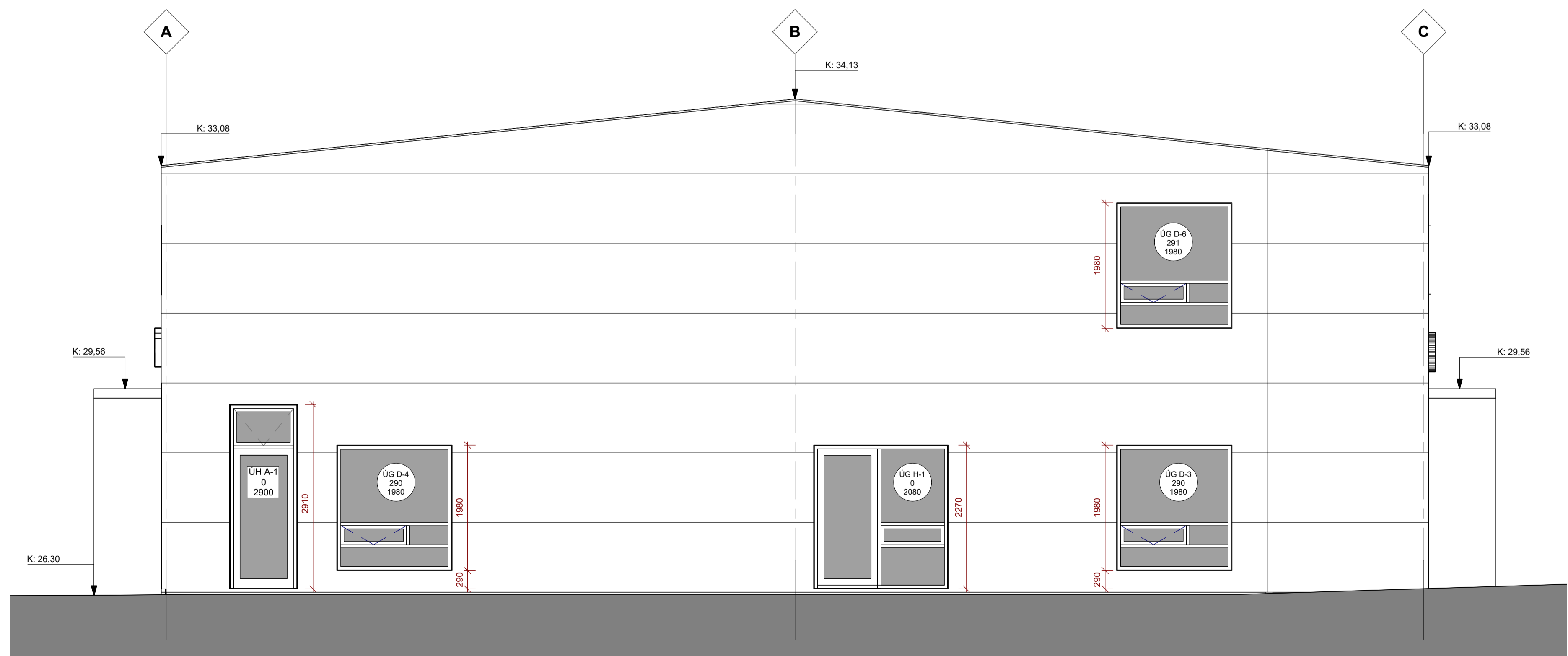
Ásýnd suður 1 : 50
